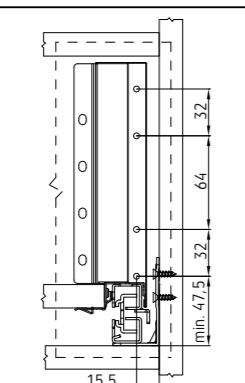
Mocowanie prowadnicy
