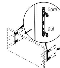
Regulacja
