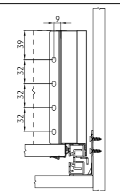
Wymiary montażowe ścianki tylnej
