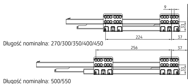
Mocowanie prowadnicy
