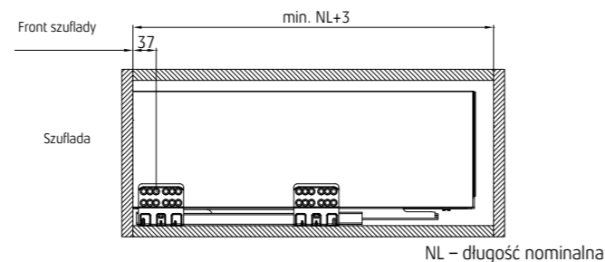
Montaż szuflady
