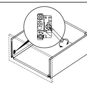
Wsunięcie szuflady
