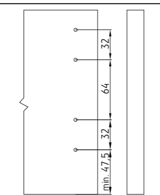
Mocowanie dystansu
