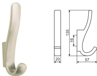
DIADEM RW07 RW07-G0006 ZnAl
