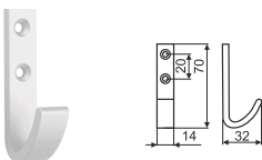
WA01 WA01-A0C00 Al
