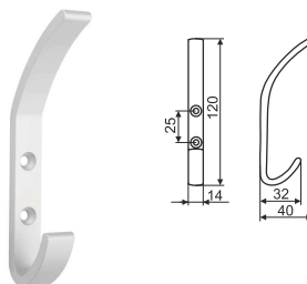
WA02 WA02-A0C00 Al
